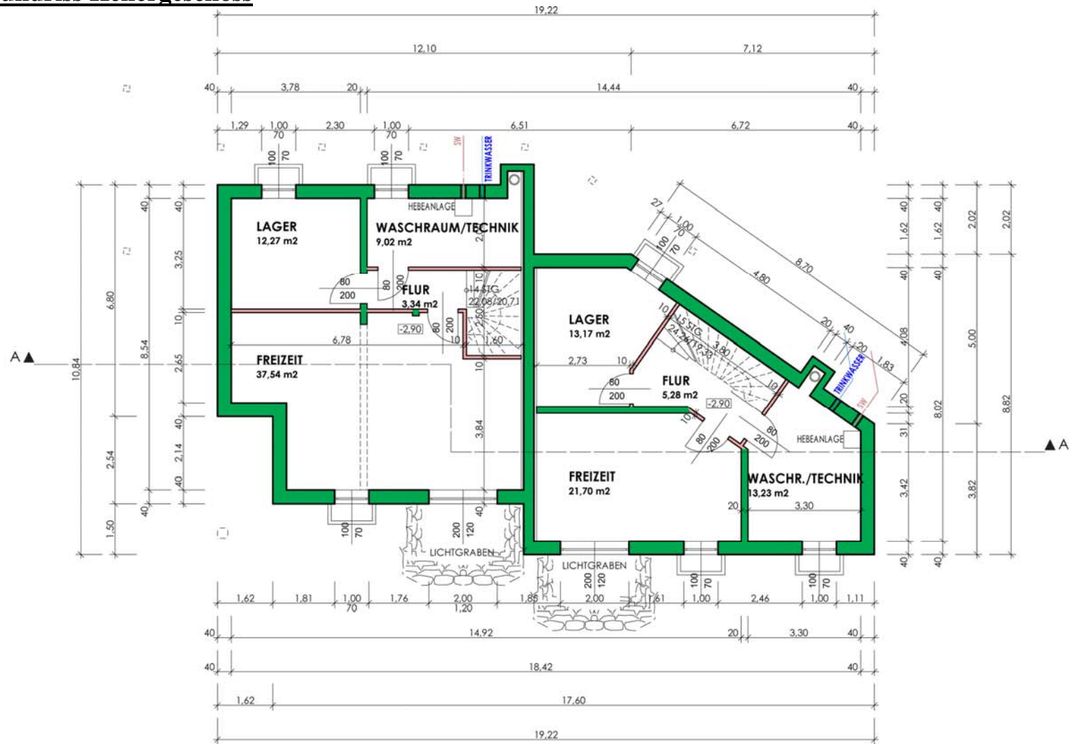
GRUNDRISS KELLERGESCHOSS
