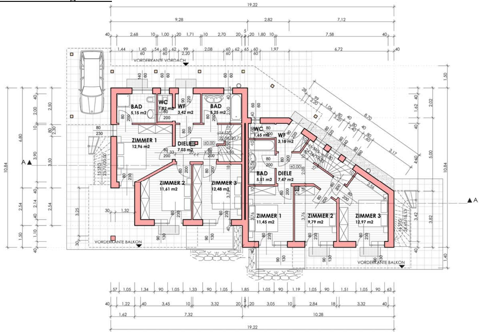
GRUNDRISS ERDGESCHOSS
